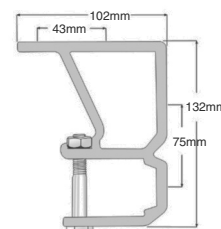
Komb. vägg / takkonsol
